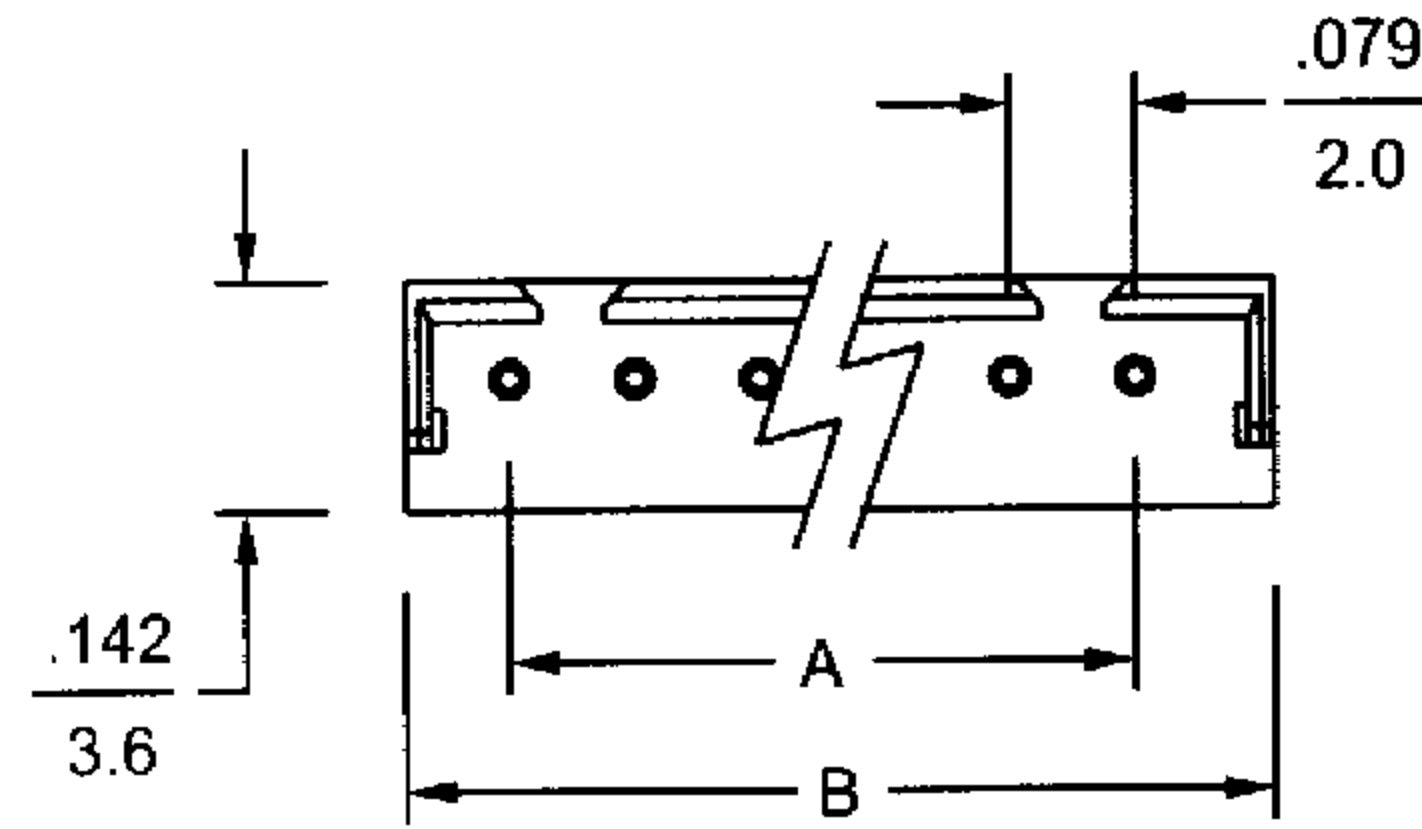
4 ~ 15 circuits
