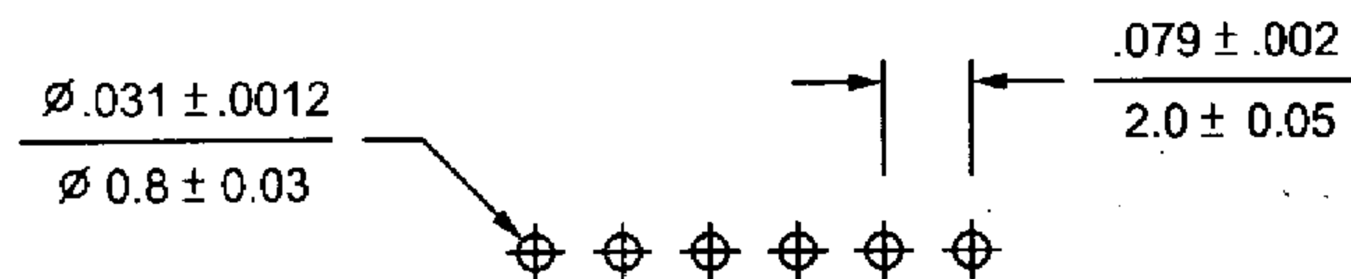
P.C.B. hole dimensions
