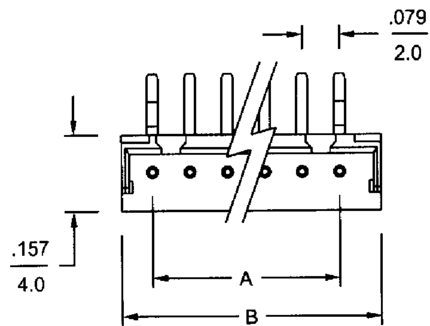
4 ~ 15 circuits
