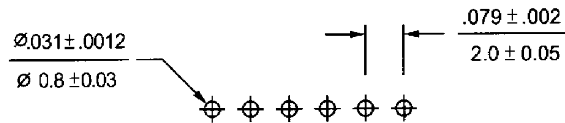
P.C.B. hole dimensions
